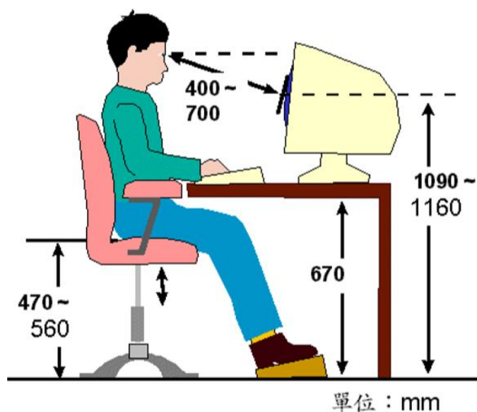
圖二 桌面高度不可調工作站參考尺寸值
