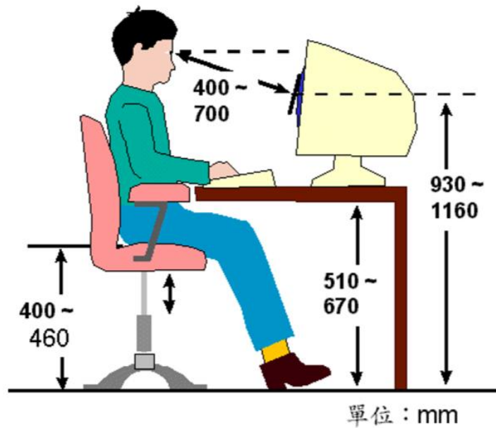
圖一 可調式工作站參考尺寸值
