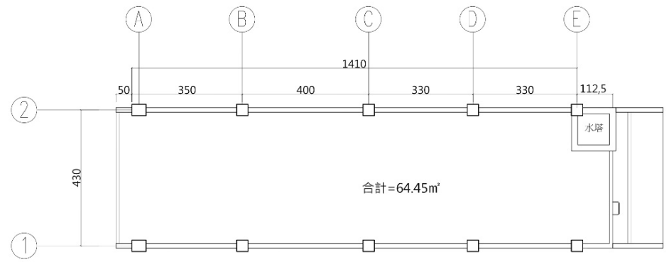
屋頂層平面圖
