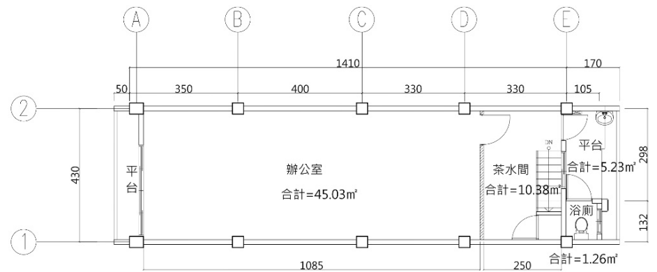
三層平面圖
